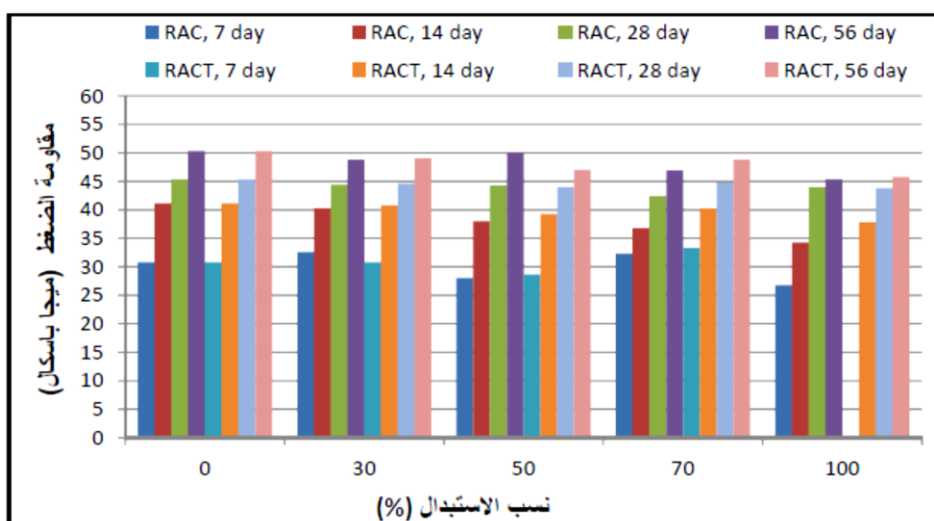
الشكل 5: مقارنة بين مقاومة الضغط للخرسانة (RAC)، والخرسانة (RACT) مع الخرسانة المرجعية (CC).
