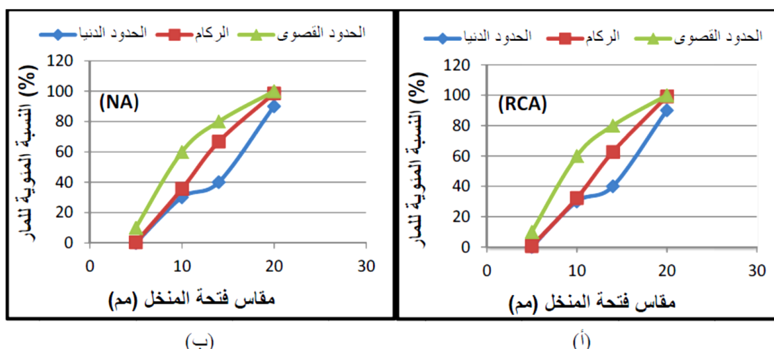
الشكل 2: منحني التدرج الحبيبي لعينة الركام الخشن. (أ) الركام المعاد تدويره، (ب) الركام الطبيعي.
